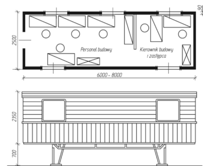
Przewoźny budynek kierownictwa budowy bez podwozia jezdnego
