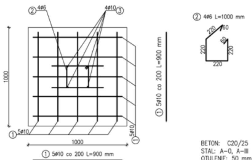
PRZEKRÓJ POZIOMY A-A - STOPY FUNDAMENTOWEJ
