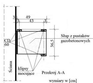
Rysunek 1. Układ i rozmieszczenie elementów rusztu
