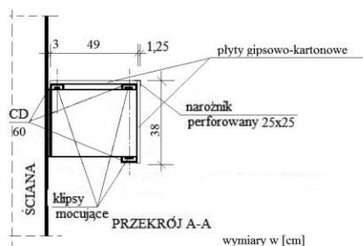
Rysunek 2. Schemat oplątowania
