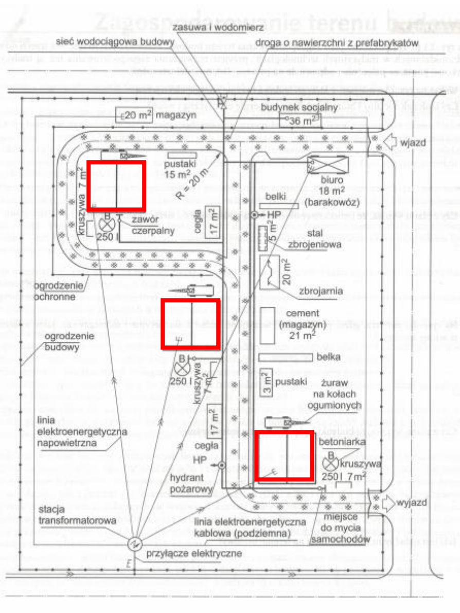
Plan zagospodarowania terenu budowy
