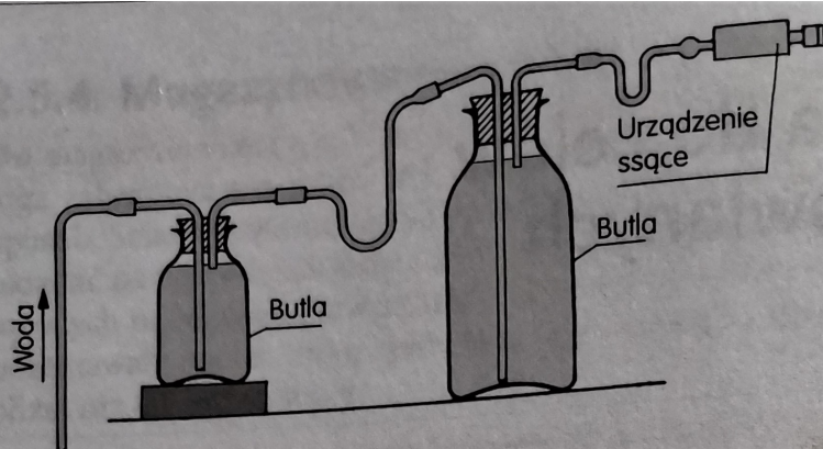
Rys. 2.9. Urządzenie do pobierania próbek wody [8]
